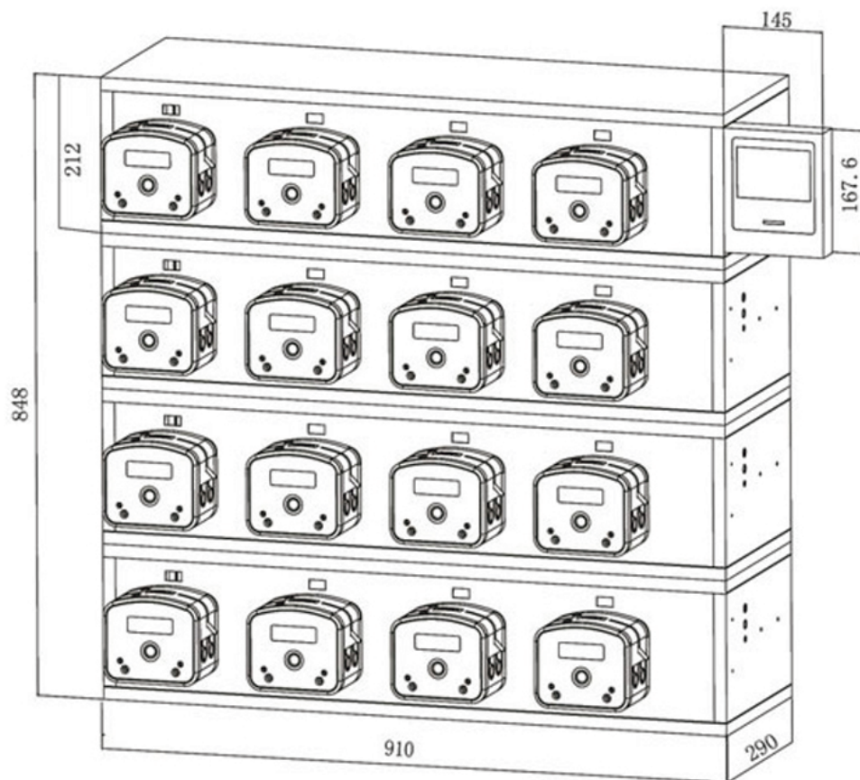
尺寸图 (单位: mm)
