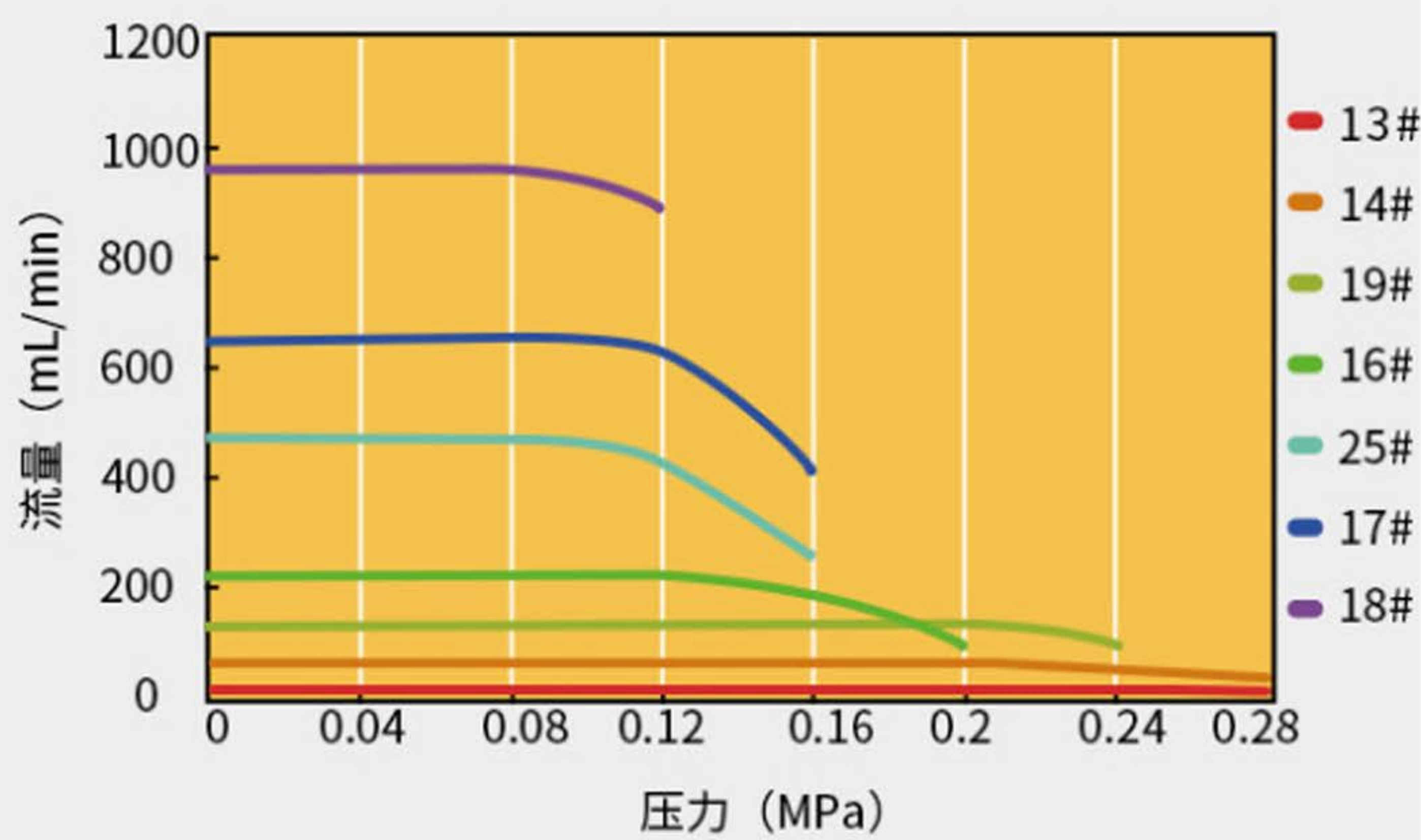
DY15泵头压力/流量曲线图 (100rpm)
