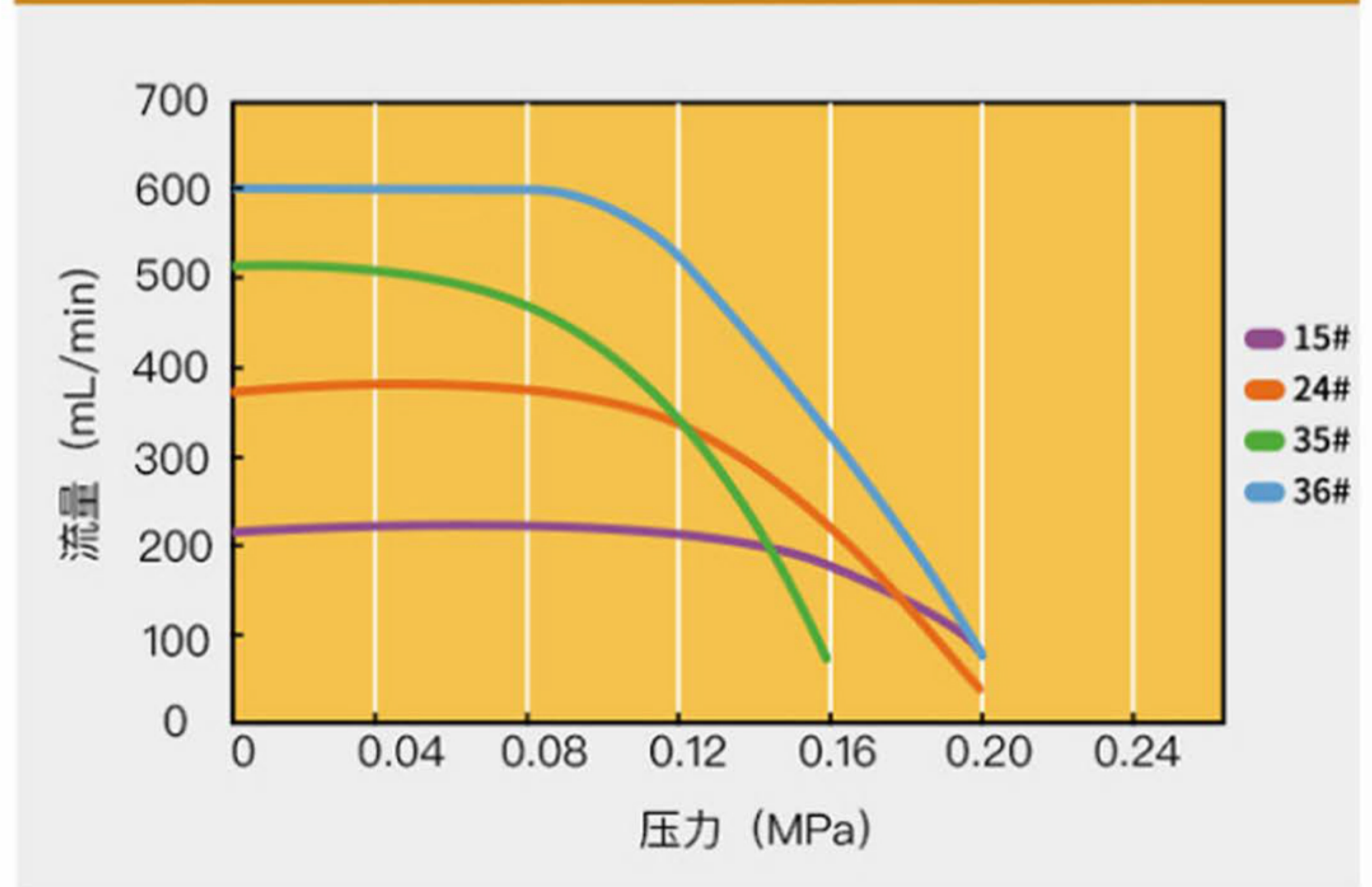
DZ25-3L泵头压力/流量曲线图 (100rpm)
