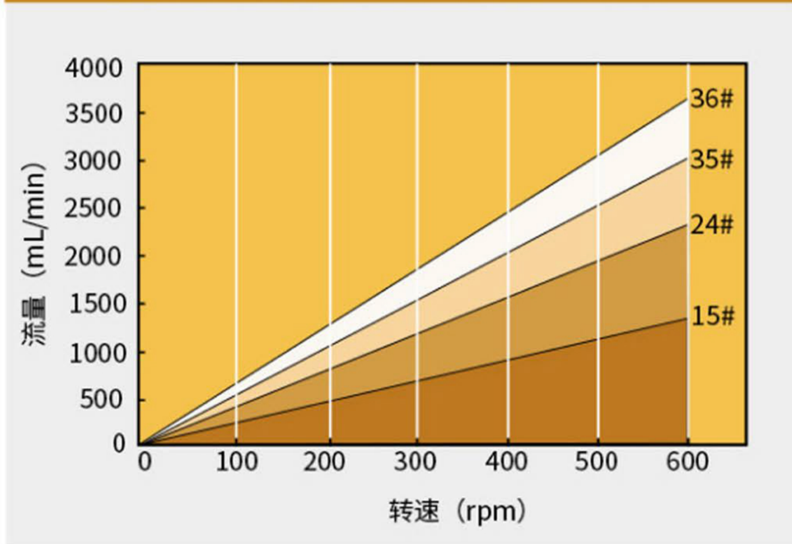
DZ25-3L泵头流量范围 (0.1-600rpm)
